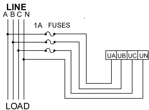
三相四线直接连接 (3LN)
