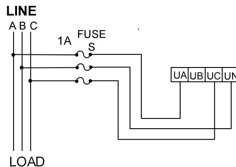
三相三线V型 (2LL)
